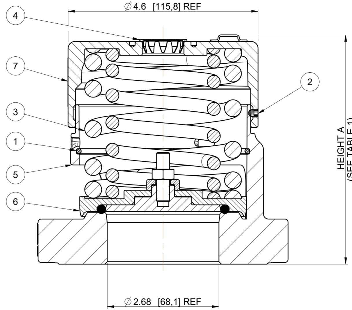
SECTION A-A
